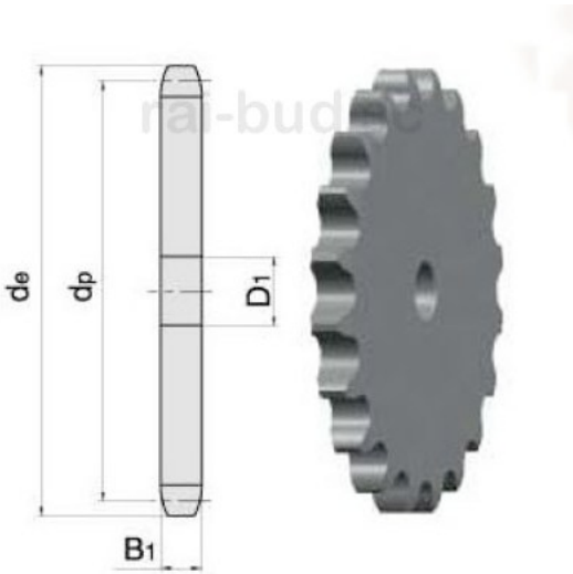
Kettenrad für Rollenketten 1", 16B, 16A
