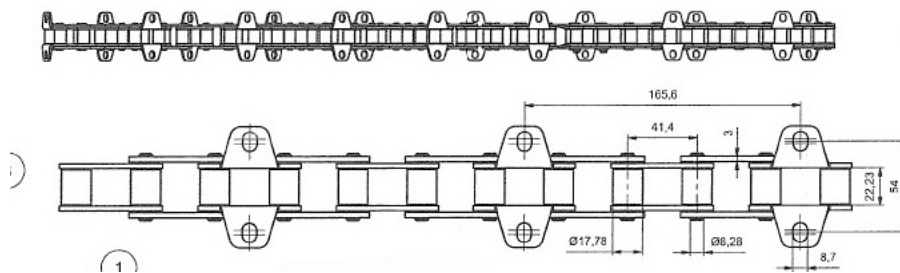
Förderkette geneigt Claas WEW 38,4VB b8,3 fi-10
