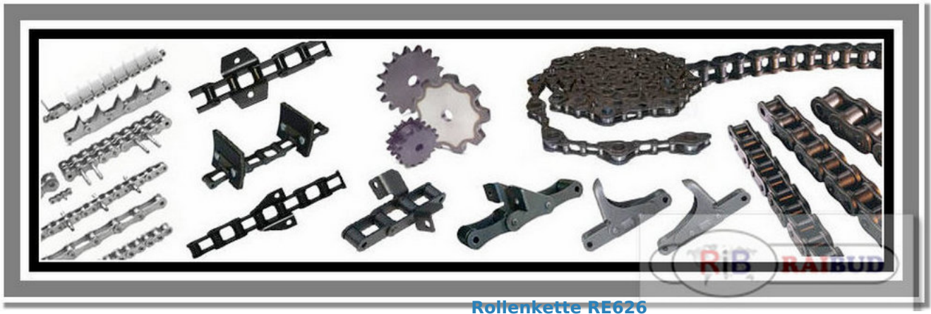
Rollenkette RE626
