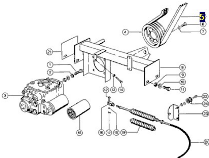
Riemen 176543.0
