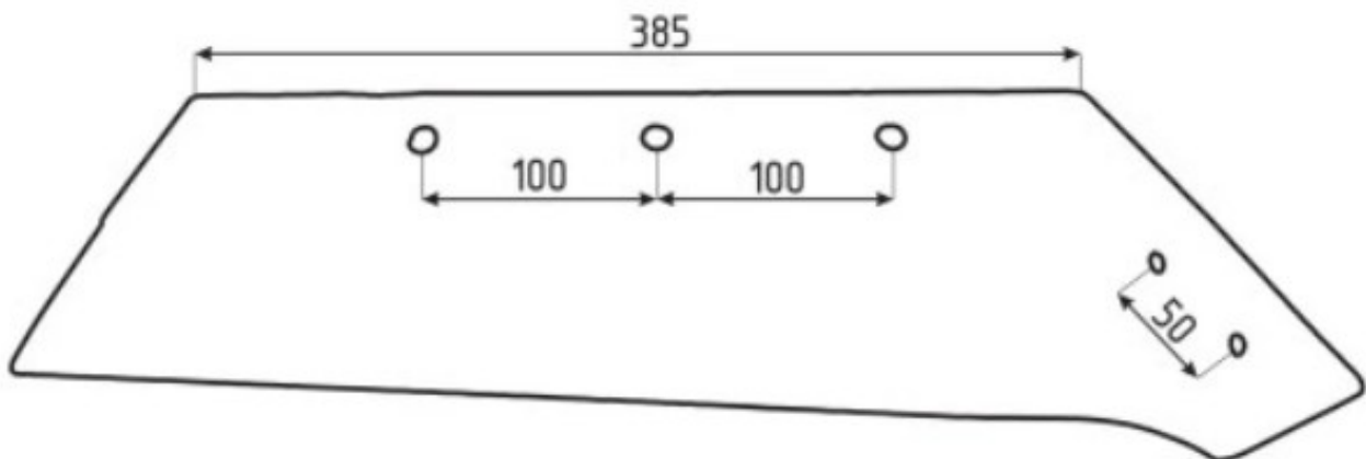
Pflugschare VN rechts WSM40 breiter PREMIUM
