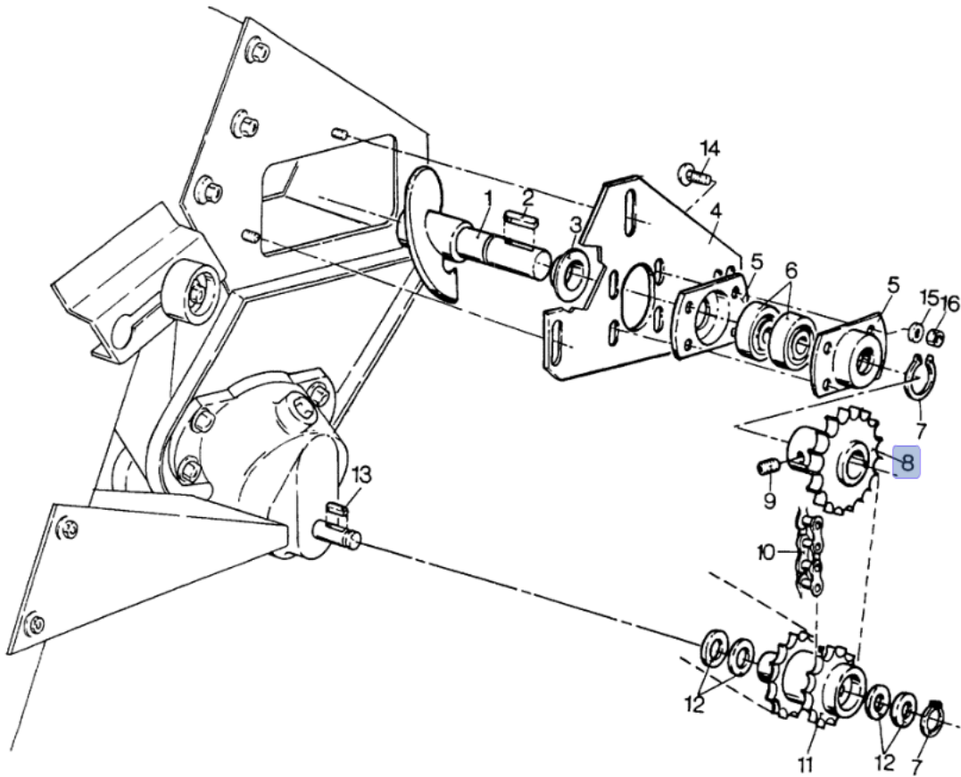
Förderkette NH 423659
