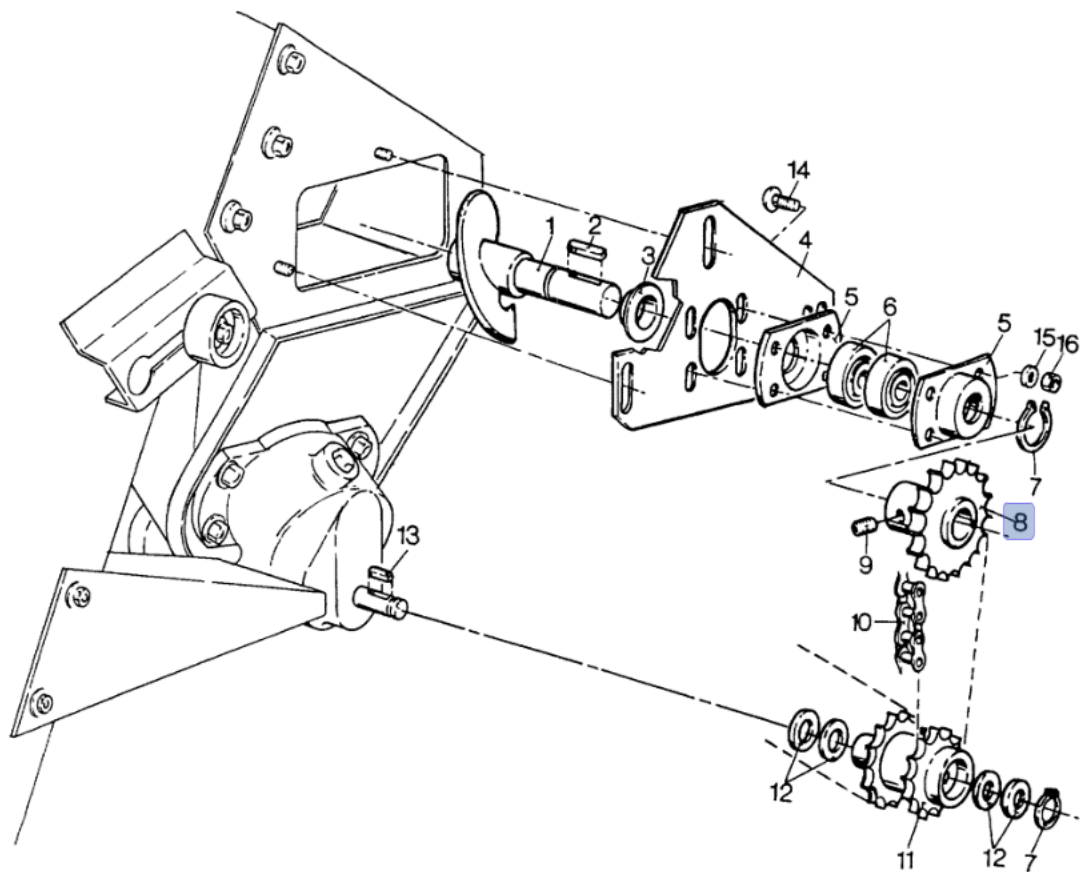
Förderkette NH 423659
