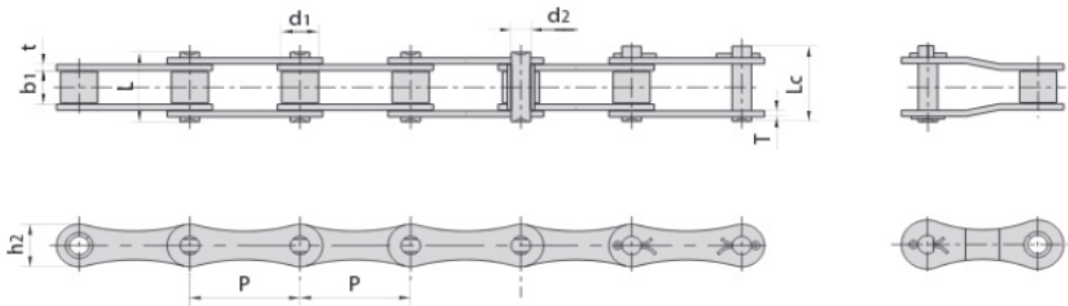
Kette 208A 2040
