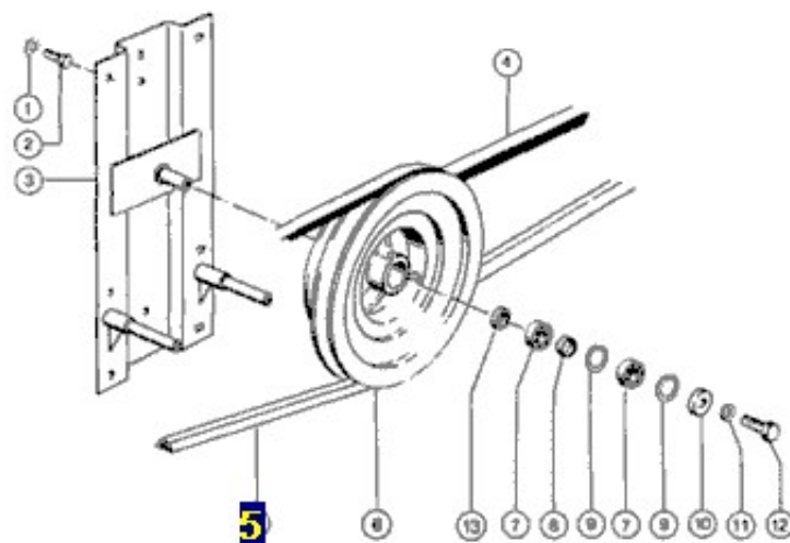
Keilriemen Claas Ersatzteil Nr. 061360.0
