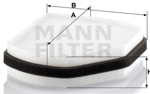
KABINENFILTER CU2897
