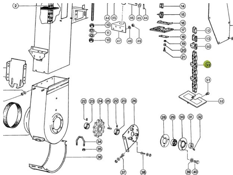
Aufzugskette Class 795362.1
