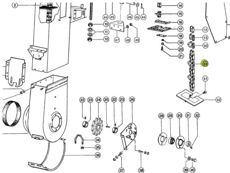
Aufzugskette Class 795362.1
