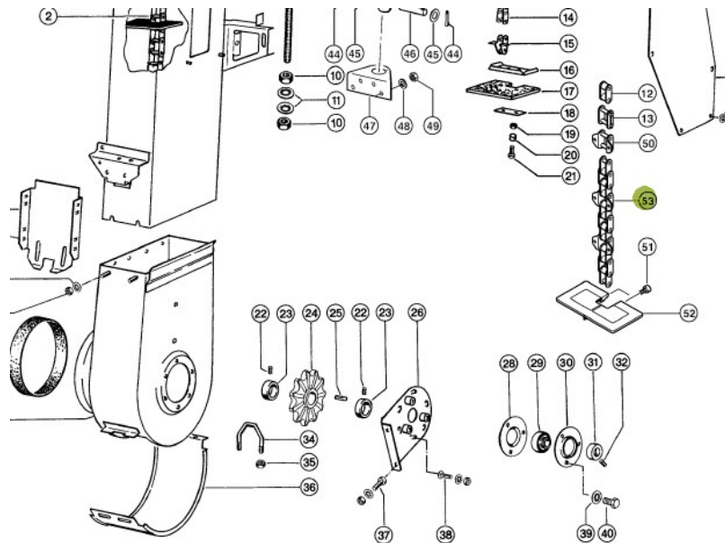
Aufzugskette Class 795362.1
