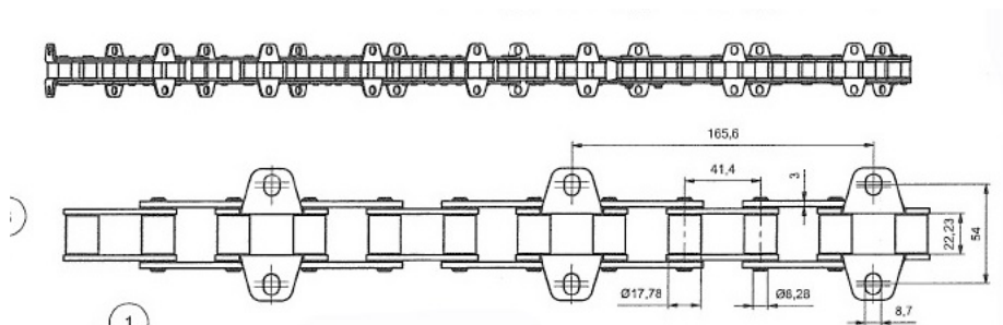
Geneigte Förderkette NEW HOLLAND 84021366 CX840 CX8070 VERSTÄRKT
