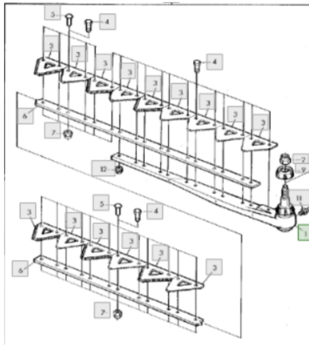
Ersatz-Mähkopf AZ41726
