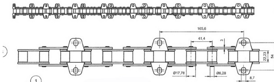
Geneigte Förderkette Claas ZEW 38.4V b7 fi-8, geneigte Förderkette Claas
