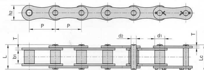
Rollenkette 1/2" 084
