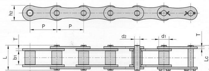
Rollenkette 1/2" 084
